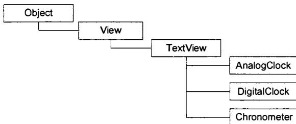
Рис. 6.20. Иерархия классов для AnalogClock, DigitalClock и Chronometer
