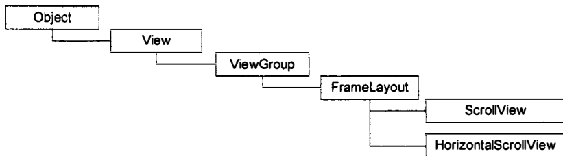
Рис. 6.4. Иерархия классов для ScrollView и HorizontalScrollView
