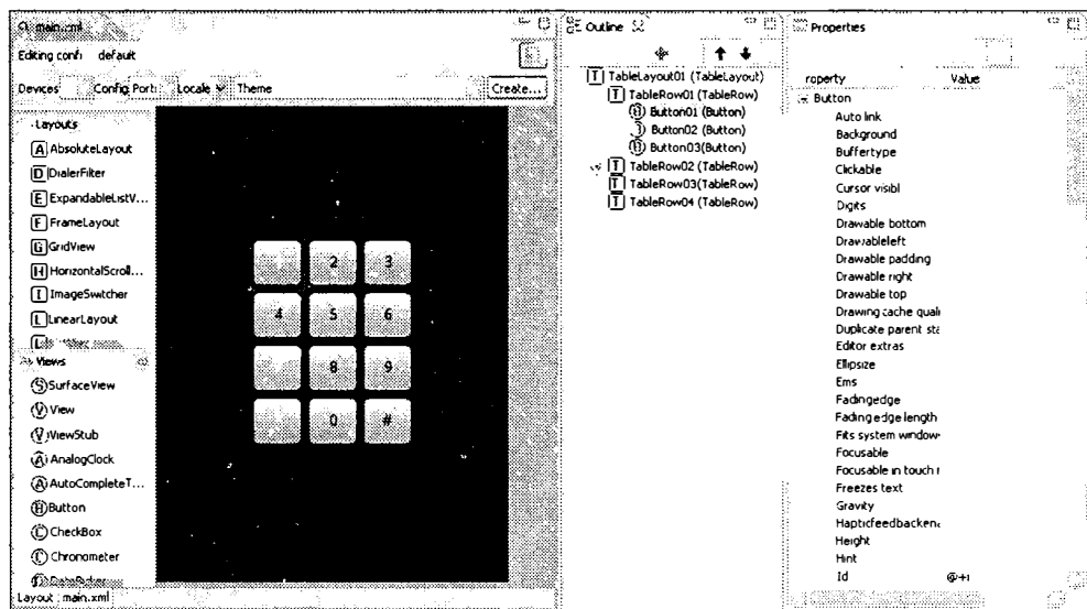
Рис. 5.3. Редактор разметки Layout Editor
