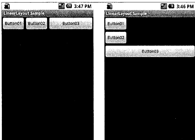
Рис. 5.6. Разметка LinearLayout с горизонтальной и вертикальной ориентациями элементов
