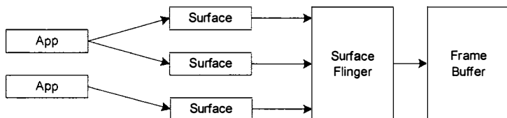
Рис. 1.2. Обработка графической информации менеджером поверхностей
