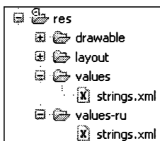
Рис. 16.7. Каталоги с локализованными строковыми ресурсами
