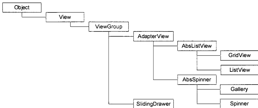
Рис. 7.4. Иерархия классов списков
