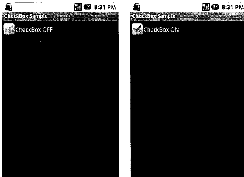
Рис. 6.11. Элемент CheckBox
