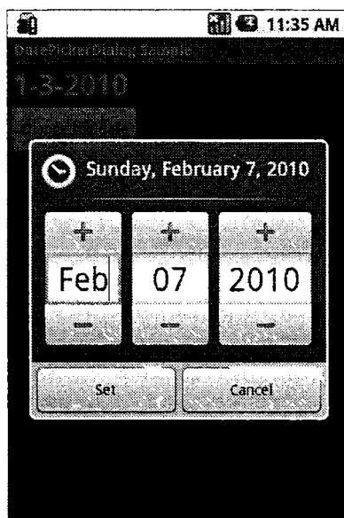
Рис. 9.8. Диалог DatePickerDialog
