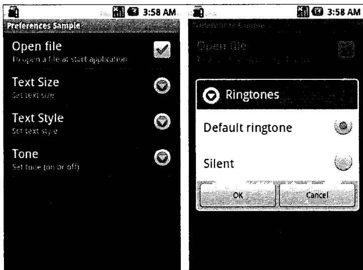
Рис. 14.8. Список RingtonePreference
