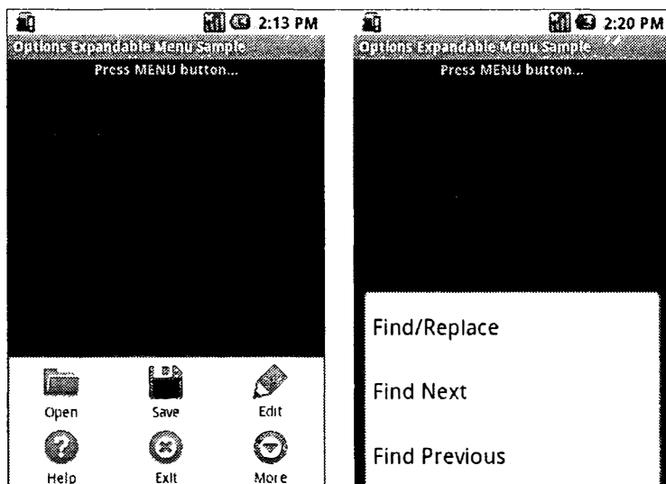
Рис. 10.3. Расширенное меню
