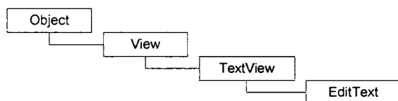
Рис. 6.1. Иерархия классов текстовых полей
