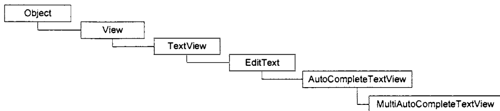
Рис. 7.1. Иерархия классов текстовых полей с автозаполнением
