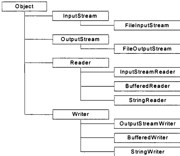
Рис. 14.1. Классы для файлового ввода-вывода в Android
