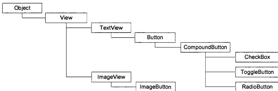
Рис. 6.7. Иерархия классов Button , CheckBox , ToggleButton , RadioButton и ImageButton
