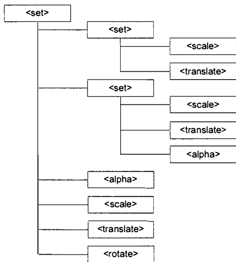
Рис. 18.2. Пример структуры XML-файла анимации
