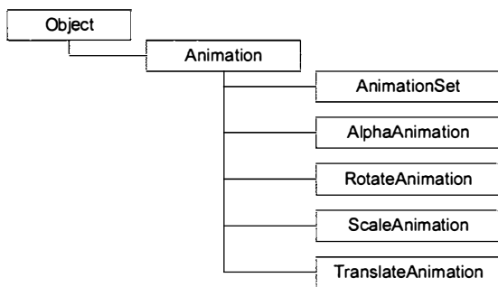
Рис. 18.1. Классы анимации в Android
