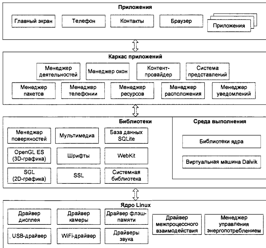
Рис. 1.1. Архитектура системы Android
