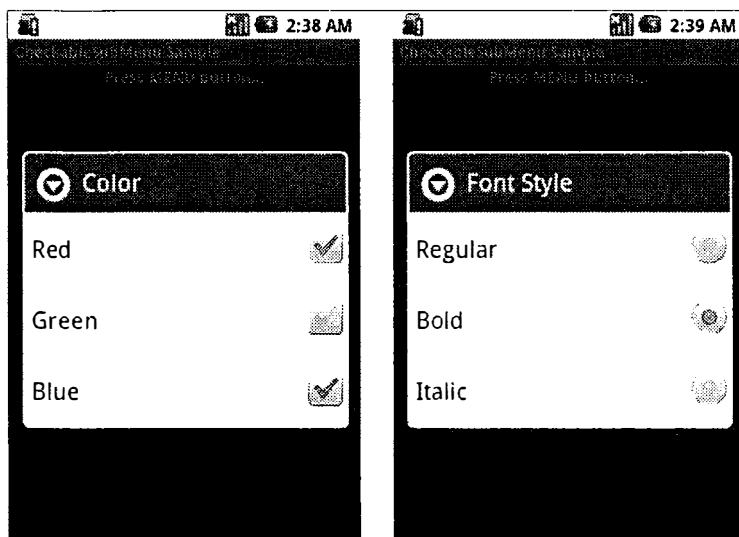
Рис. 10.6. Группы подменю с флажками и радиокнопками
