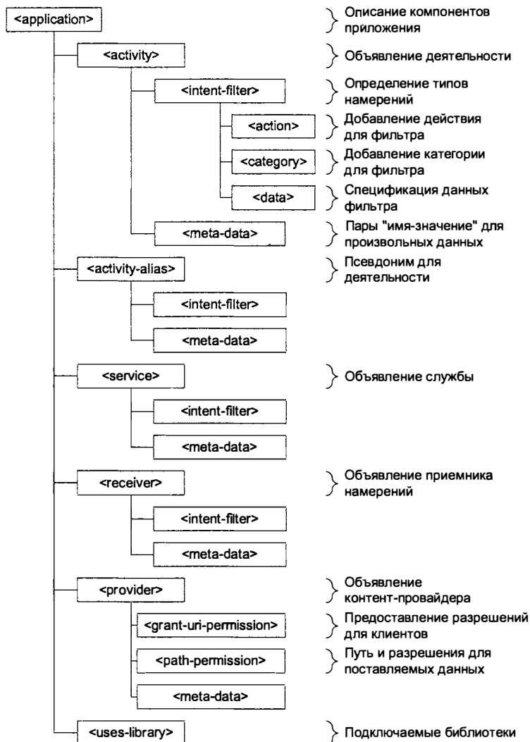
Рис. 4.4. Структура элемента <application>
