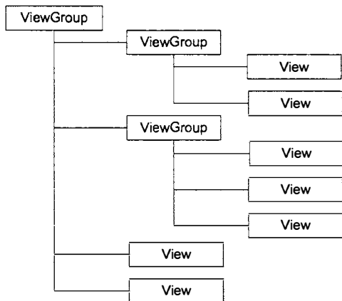
Рис. 5.2. Пример дерева представлений для деятельности
