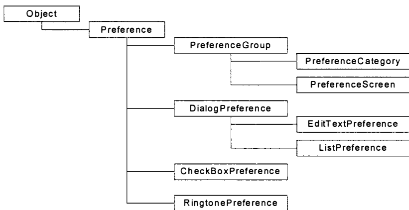
Рис. 14.4. Иерархия классов предпочтений
