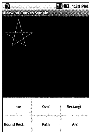
Рис. 17.5. Рисование графических объектов на канве
