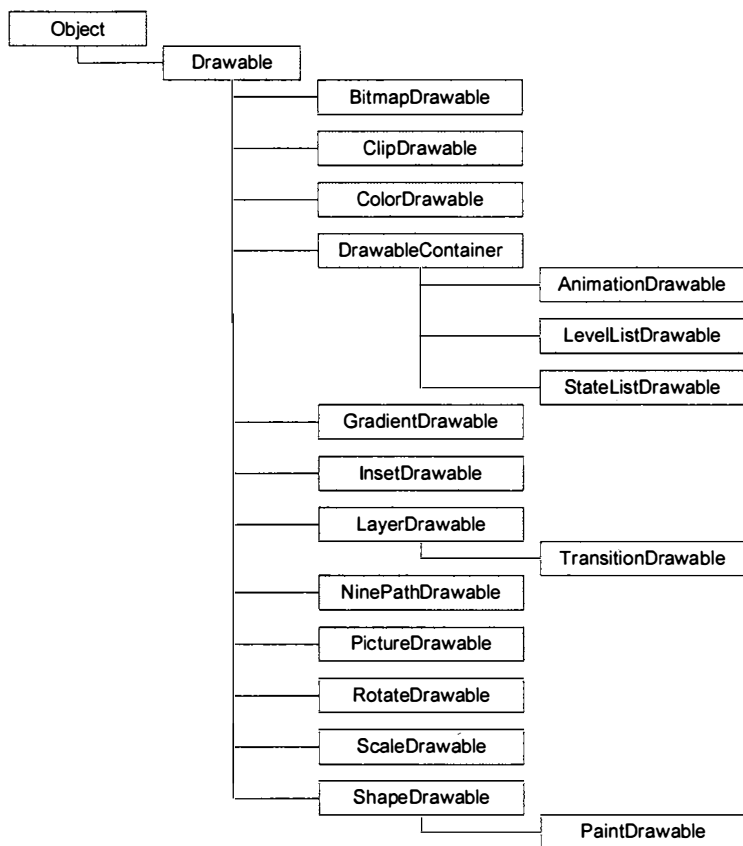
Рис. 17.1. Иерархия графических классов
