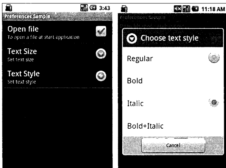
Рис. 14.7. Использование ListPreference для выбора стиля текста
