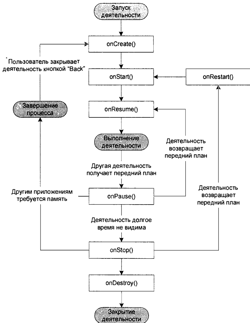
Рис. 11.1. Жизненный цикл деятельности
