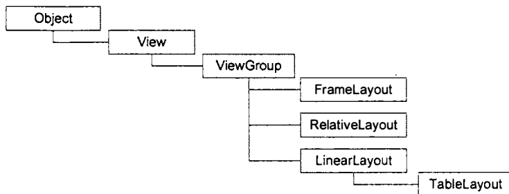
Рис. 5.4. Иерархия классов разметок
