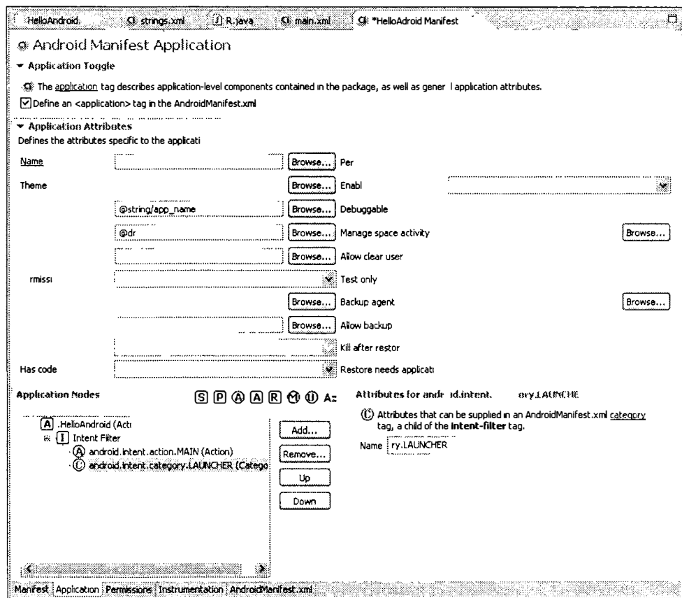
Рис. 4.2. Редактор файла манифеста
