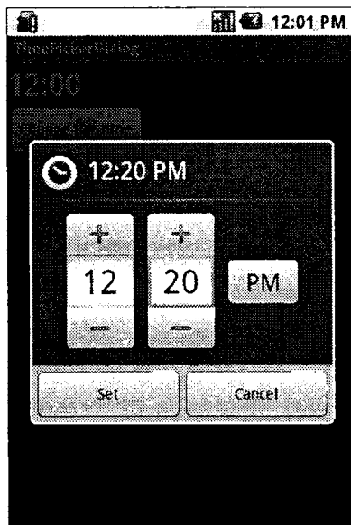
Рис. 9.9. Диалог TimePickerDialog
