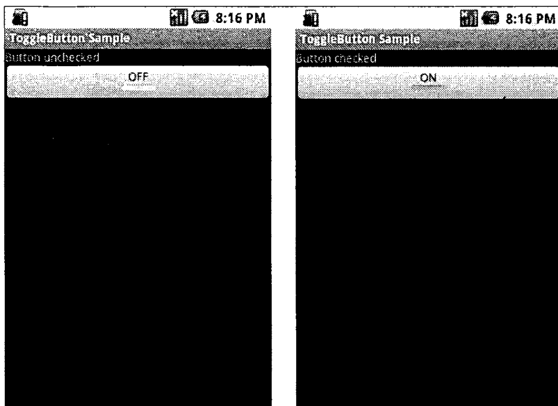
Рис. 6.12. Элемент ToggleButton
