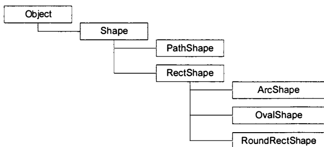
Рис. 17.3. Иерархия классов графических примитивов
